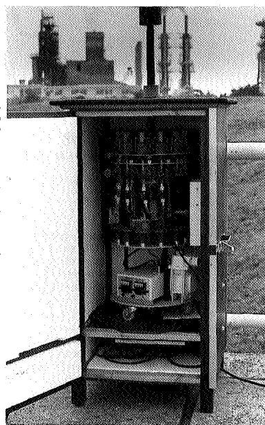
Opstelling voor metingen van luchtvervuiling
