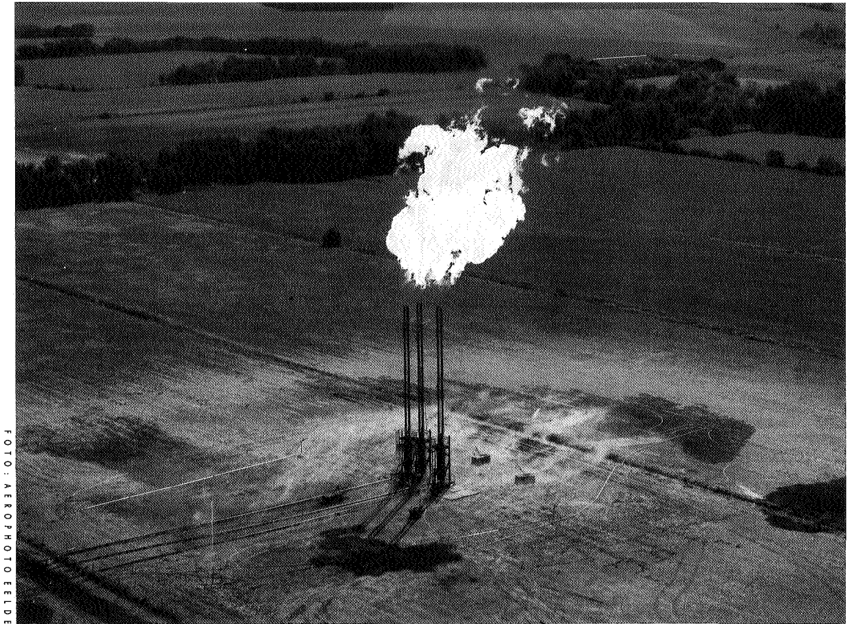
Affakkelen van een gasput bij Langelo
